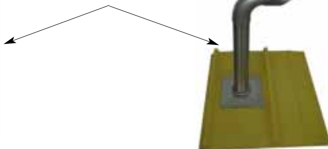
Рис. 34 На фото выше приведен фрагмент стыкового соединения дымохода и воздуховода (от прибора PANRAD) на кровле из профнастила. Каждое такое соединение выполняется по размерам с последующей гидроизоляцией.
