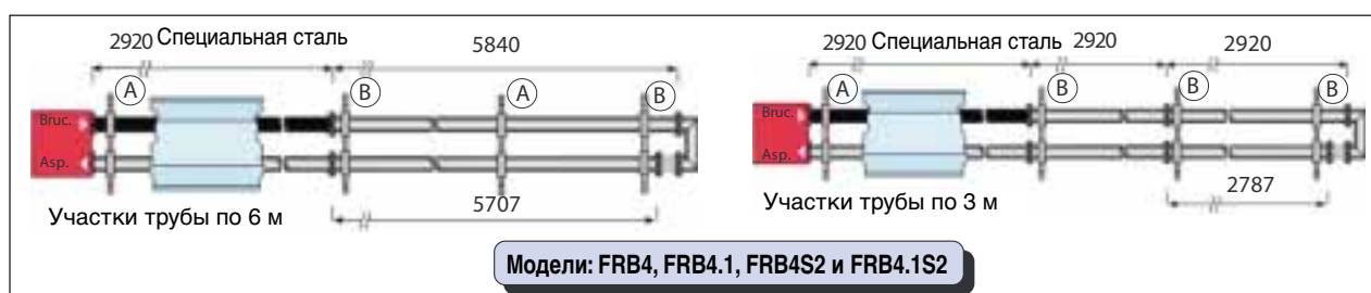
Рис.21 Схема сборки нагревательных панелей длиной 6 метров
